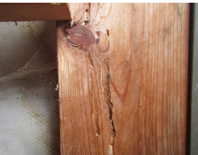
スギノアカネトラカミキリに加害された柱
